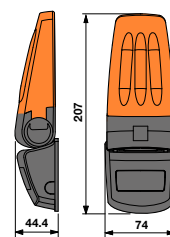
APPLICAZIONE A PARETE
