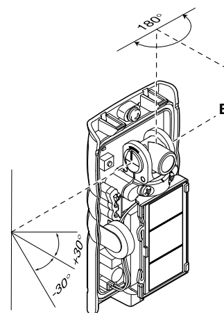
OTTICA ORIENTABILE
