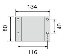
BASE DI FISSAGGIO CODICE DI RICAMBIO 999626
