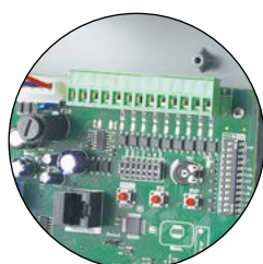
INGRESSI OPTOISOLATI CON SEGNALAZIONE A LED
