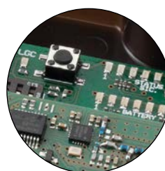
8 LED ROSSI STATO SICUREZZA 8 LED VERDI LIVELLO CARICA- BATTERIA
