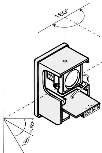
OTTICA ORIENTABILE
